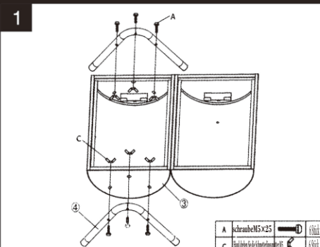
Installationsabschlussdiagramm
